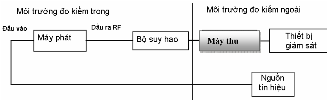
Hình 3. Cấu hình đo kiểm cho máy phát
