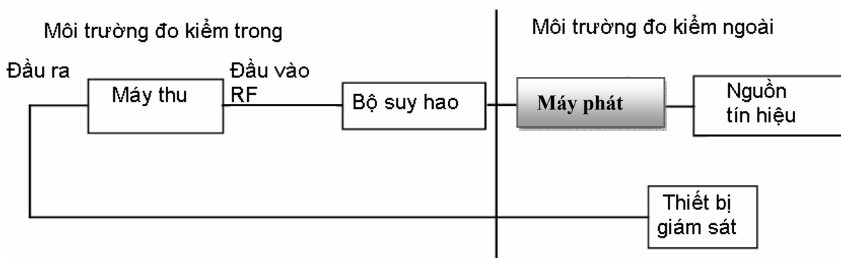
Hình 4. Cấu hình đo kiểm cho máy thu
